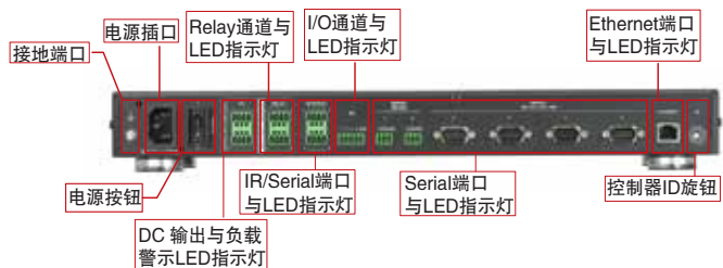
• VK2100 后视图
