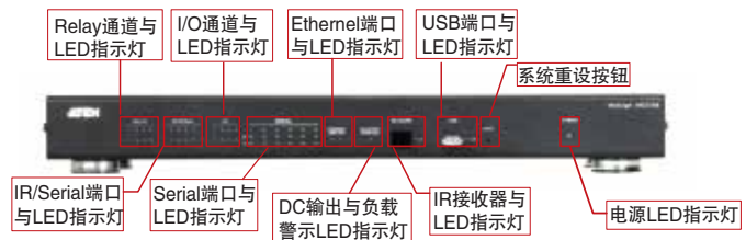
• VK2100 前视图
