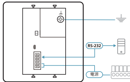
背視圖
