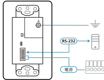
背視圖
