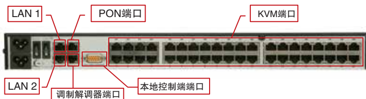
• KN2140v 后视图
